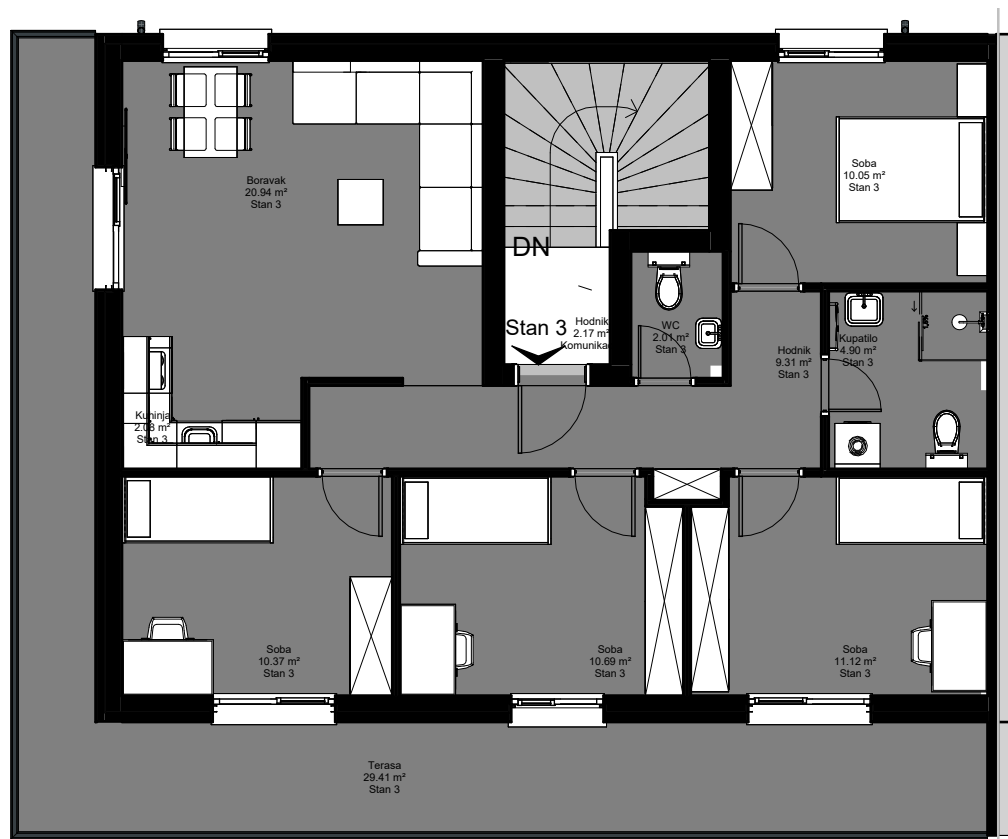
1 C02 - Potkrovlje - Položaj stana 3 na osnovi 1 : 100
